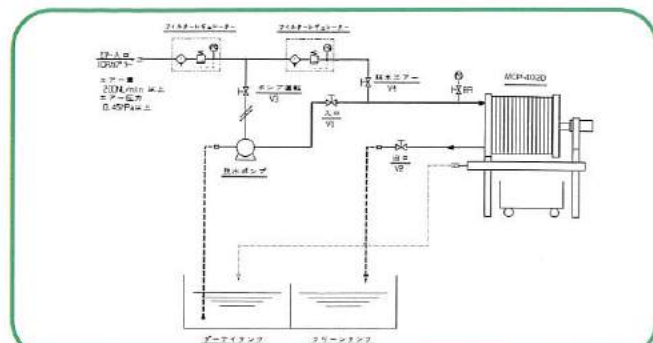
カスポンプレスフローシート図
