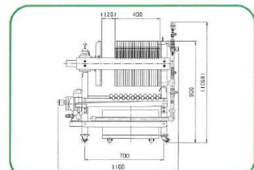
カスポンプレス外観図 (MCP4020型)
